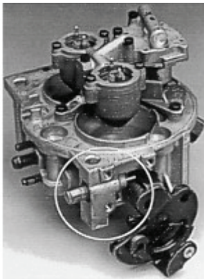
Fig. 20: „Smart idle screw“ (prototype [20])
